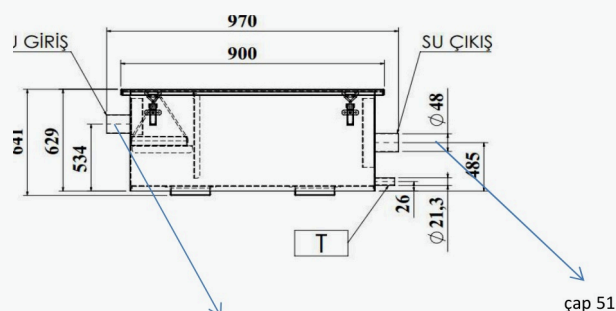
VUE LATÉRALE
